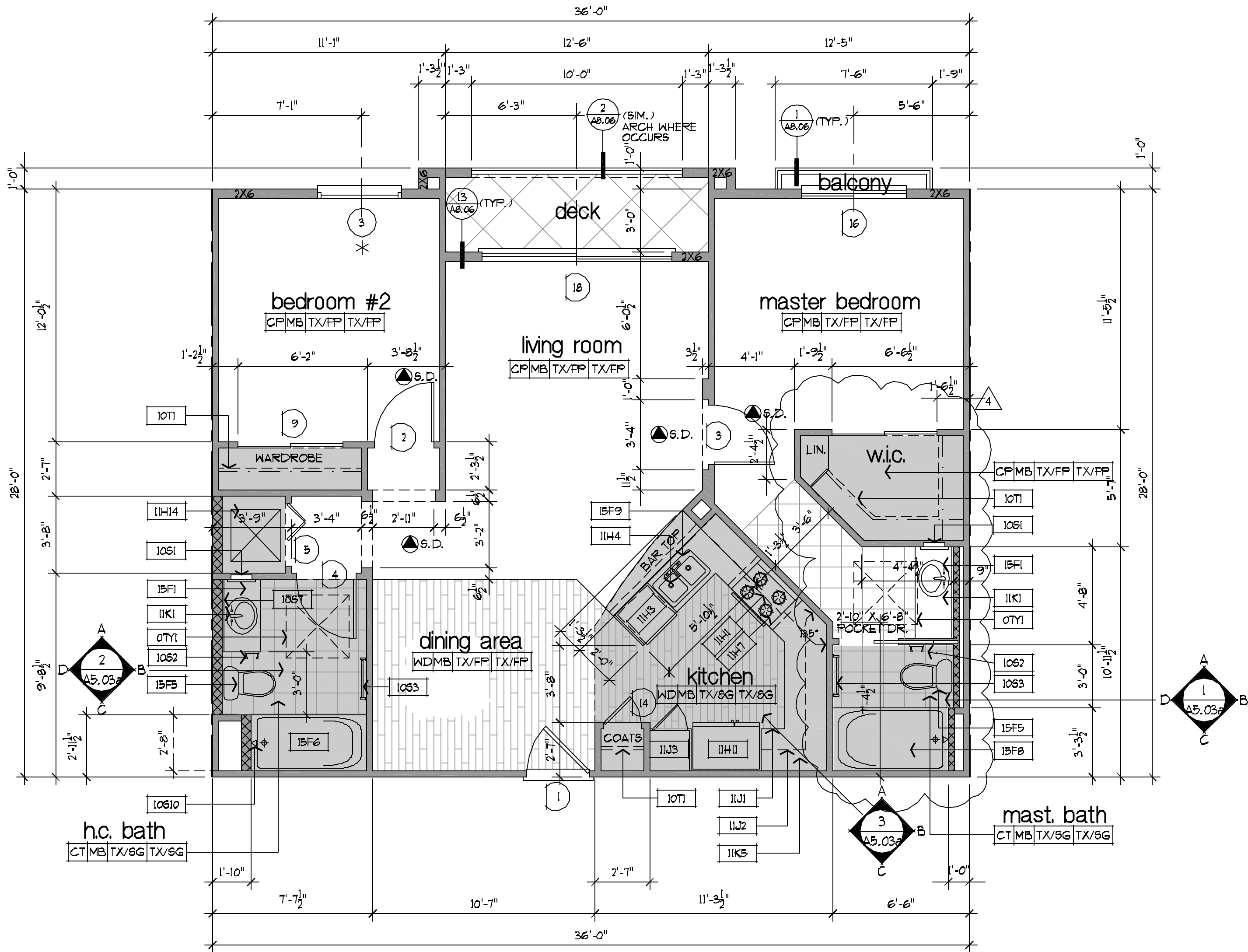
unit C SCALE: 1/4" = 1'-0"
