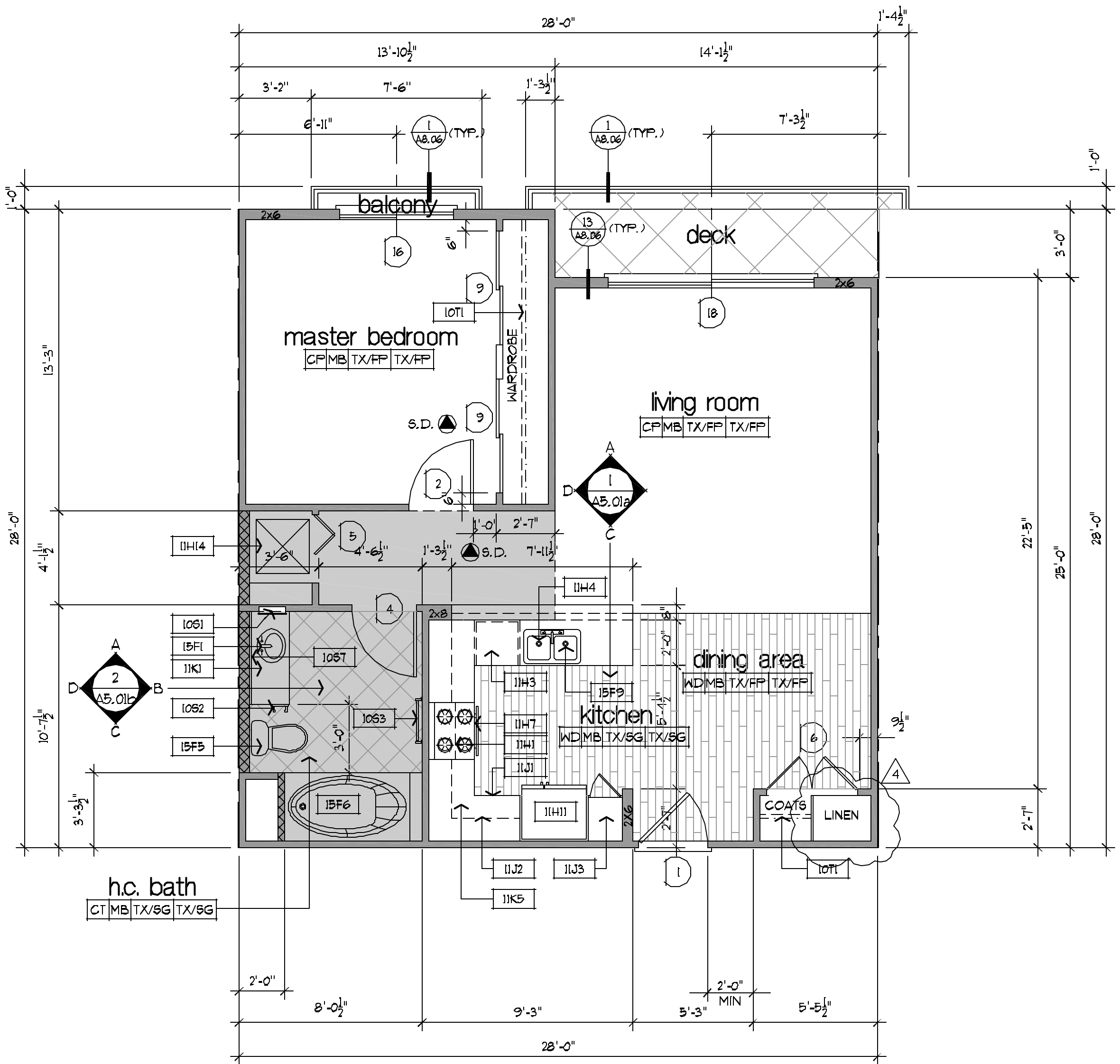
unit A SCALE: 1/4" = 1'-0"
